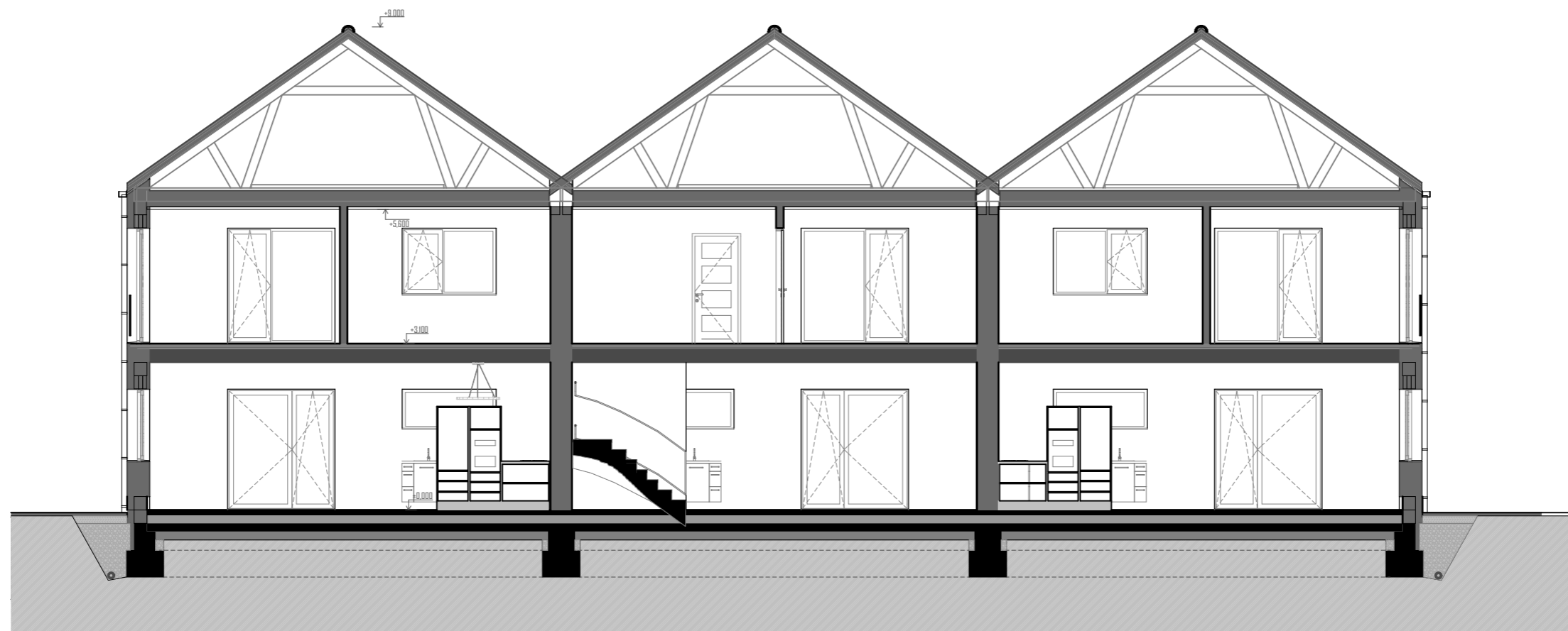
ŘEZ PŘÍČNÝ
